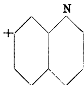
Cleve.
